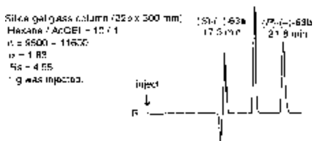
図10 M \alpha NP acid menthol esters の HPLC 分離
