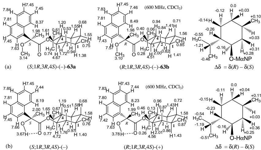
図 11 MαNP および HαNP acid menthol esters の NMR データ
