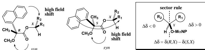
図 12 M\alpha NP esters の優先安定立体配座と NMR \Delta\delta 値のセクター則
