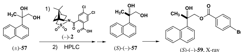
図6 2-(1-naphthyl)propane-1,2-diol ( 57 )の光学分割と絶対配置の決定
