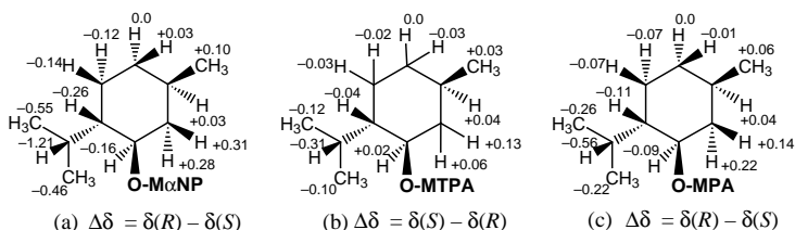
図 13 各キラルカルボン酸エステルの NMR \Delta\delta 値の比較
