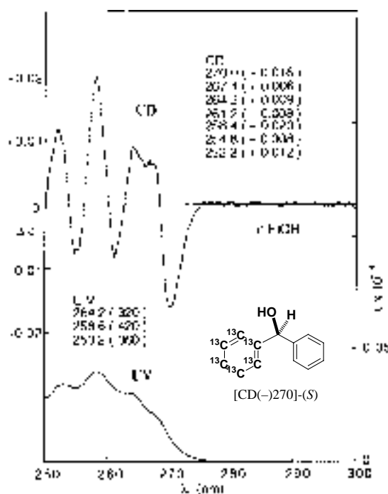
図5 (S)- \alpha -phenylbenzene(1,2,3,4,5,6- 13 C 6 )methanol( 43 )のエタノール中におけるUVとCDスペクトル
