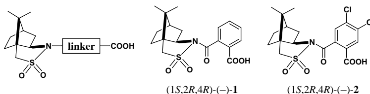
図3 2,10-camphorsultam 部分を含んだ新規キラルカルボン酸の分子設計
