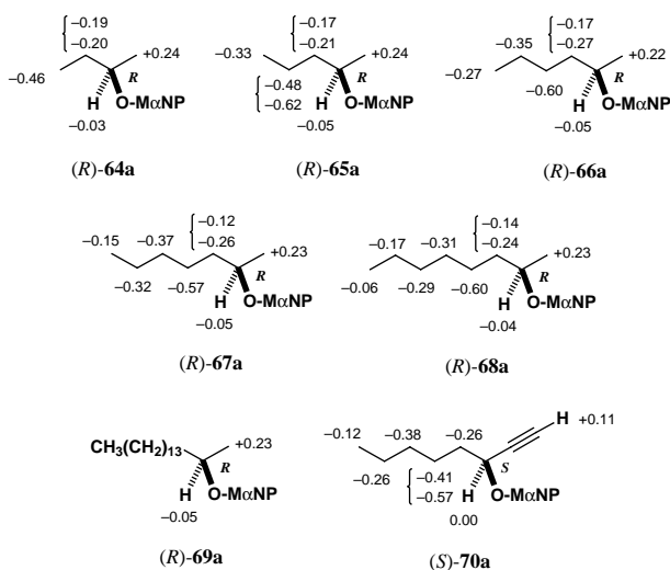
図 17 (S)-(+)-MαNP acid を用いた NMR \Delta\delta 法による第一溶出成分のアルコール部分の絶対配置決定: 実測 \Delta\delta 値
