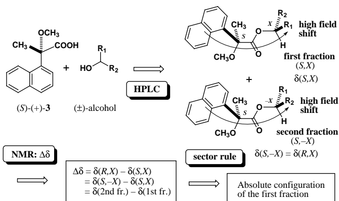
図 16 アルコールの (S)-(+)-MαNP による光学分割と NMR \Delta\delta 法による第一溶出成分の絶対配置決定
