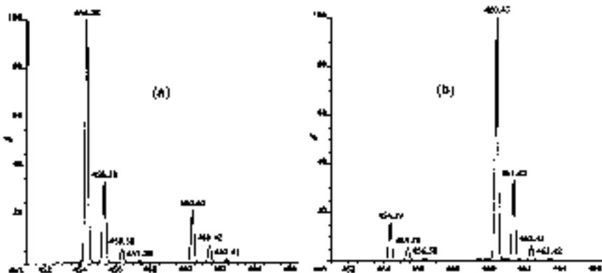
図 23 2-hexadecanol (69.77% ee) M \alpha NP エステルの MS スペクトル: JEOL, JMS GCmate II, EI 40 eV; (a) 第一溶出成分, (S,R)-72 と (R,S)-72- d 6 を含む; (b) 第二溶出成分, (S,S)-72 と (R,R)-72- d 6 を含む。
