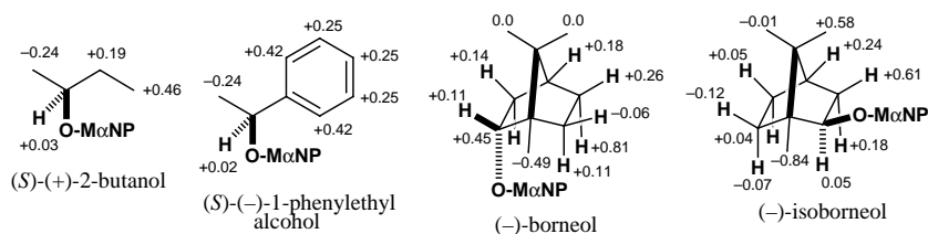
図 14 M\alpha NP acid 法による NMR \Delta\delta 値と絶対配置
