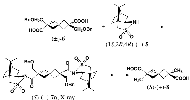
図2 カルボン酸(6)の光学分割, X線結晶解析による絶対配置の決定 および光学的に純粋な Fecht 酸類縁体の合成
