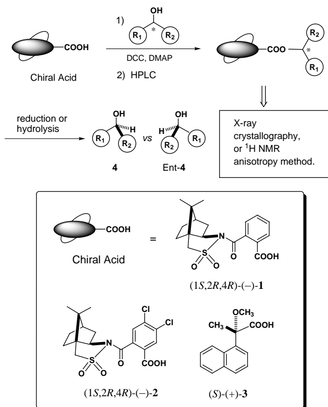
図1 キラルカルボン酸を用いたアルコール類の光学分割と絶対配置の決定
